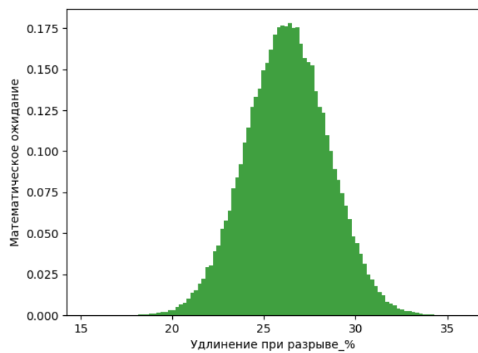
Рисунок 15. Нормальное распределение результатов измерения деформации нити
