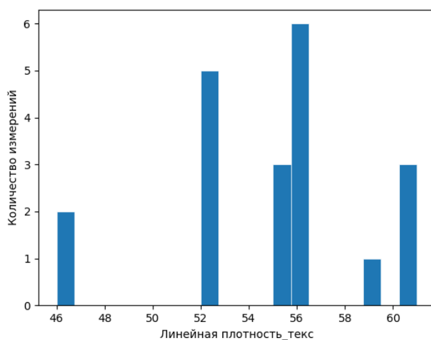
Рисунок 7. Распределение результатов расчета линейной плотности нити
