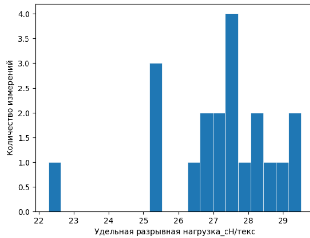
Рисунок 10. Распределение результатов измерения удельной разрывной нагрузки
