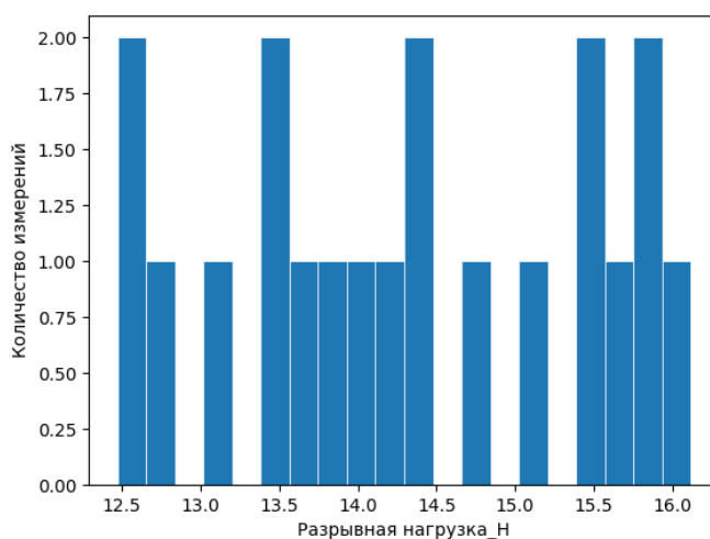
Рисунок 8. Распределение результатов измерения силы разрыва нити
