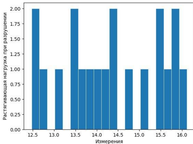
Рисунок 7. Растягивающая нагрузка при разрушении
