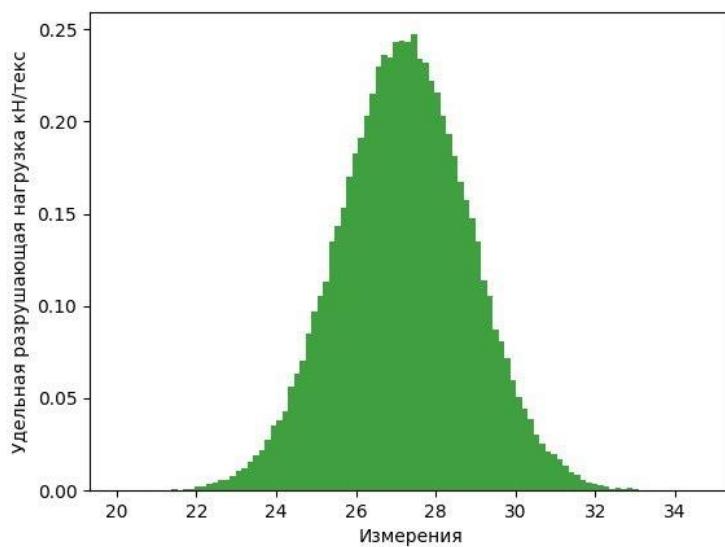
Рисунок 11. Удельная разрушающая нагрузка кН\текс
