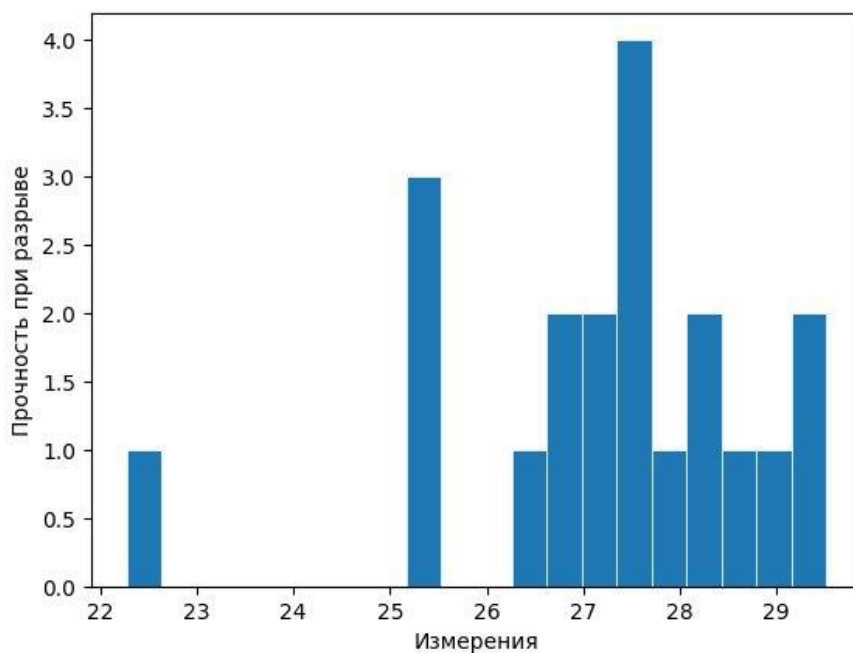
Рисунок 5. Прочность при разрыве нити.
