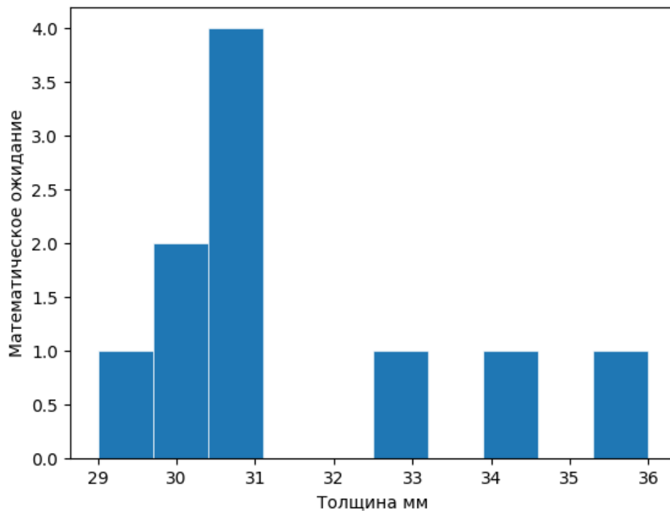
Рисунок 5 Распределение результатов измерения нити, мм
