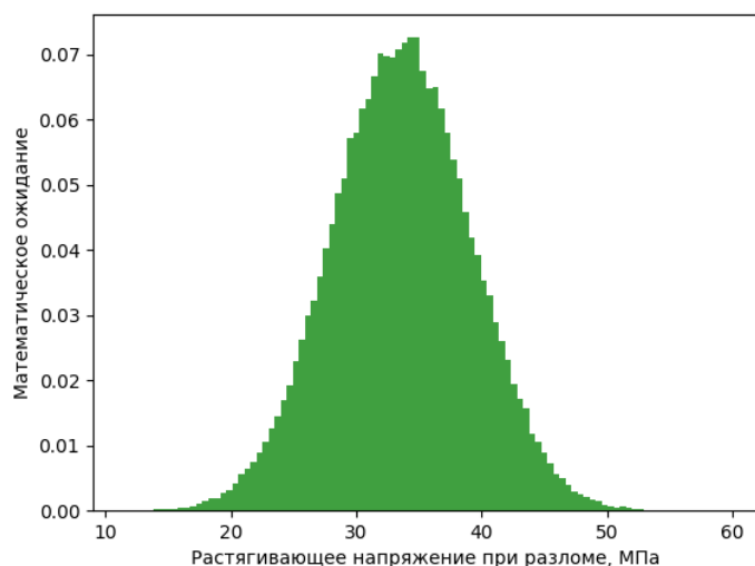
Рисунок 12 Нормальное распределение результатов измерения растягивающего напряжения
