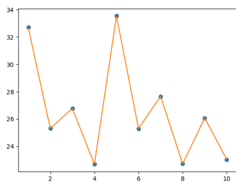
Рисунок 2 Сила разрыва нити, Н
