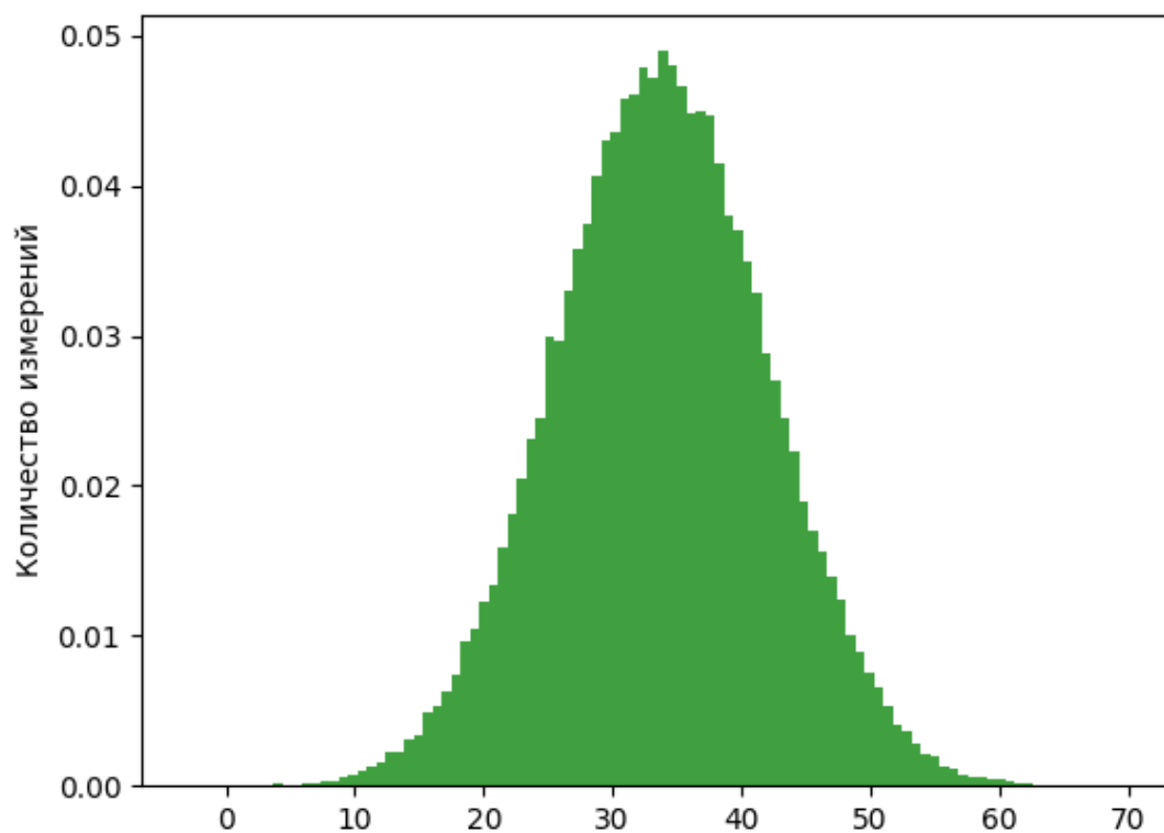
Рисунок 10. Нормальное распределение результатов измерения силы разрыва нити
