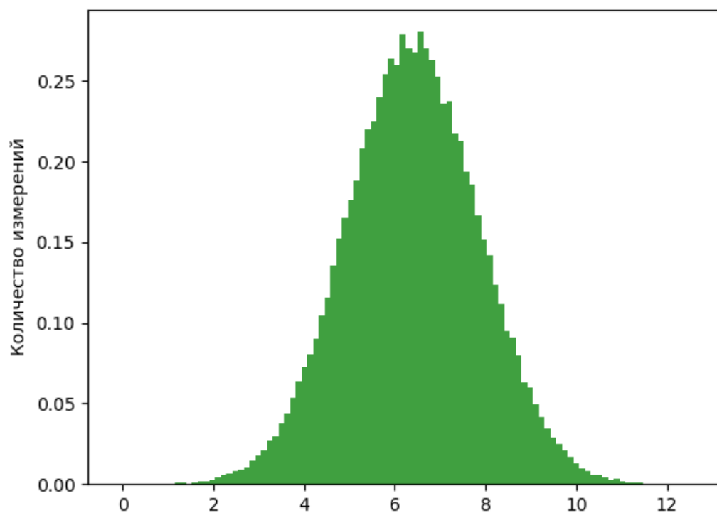
Рисунок 11. Нормальное распределение результатов измерения деформации нити
