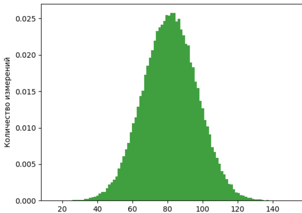
Рисунок 12. Нормальное распределение результатов измерения растягивающего напряжения
