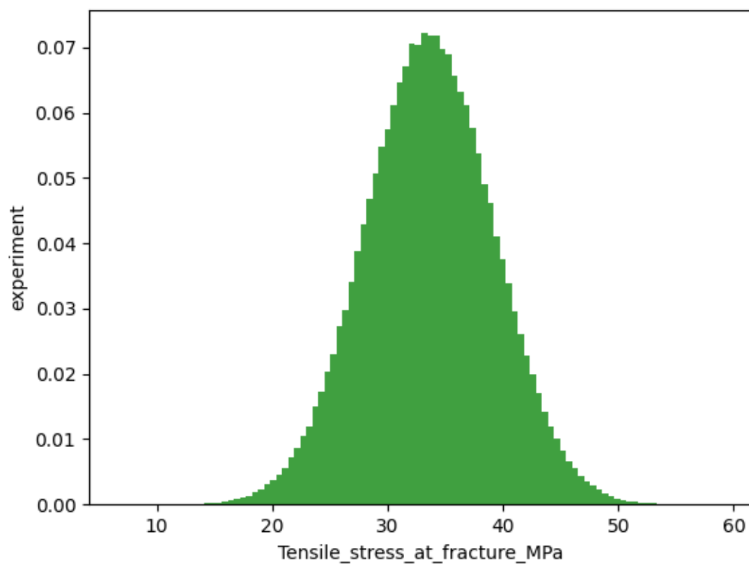
Рисунок 10. Нормальное распределение результатов измерения растягивающего напряжения
