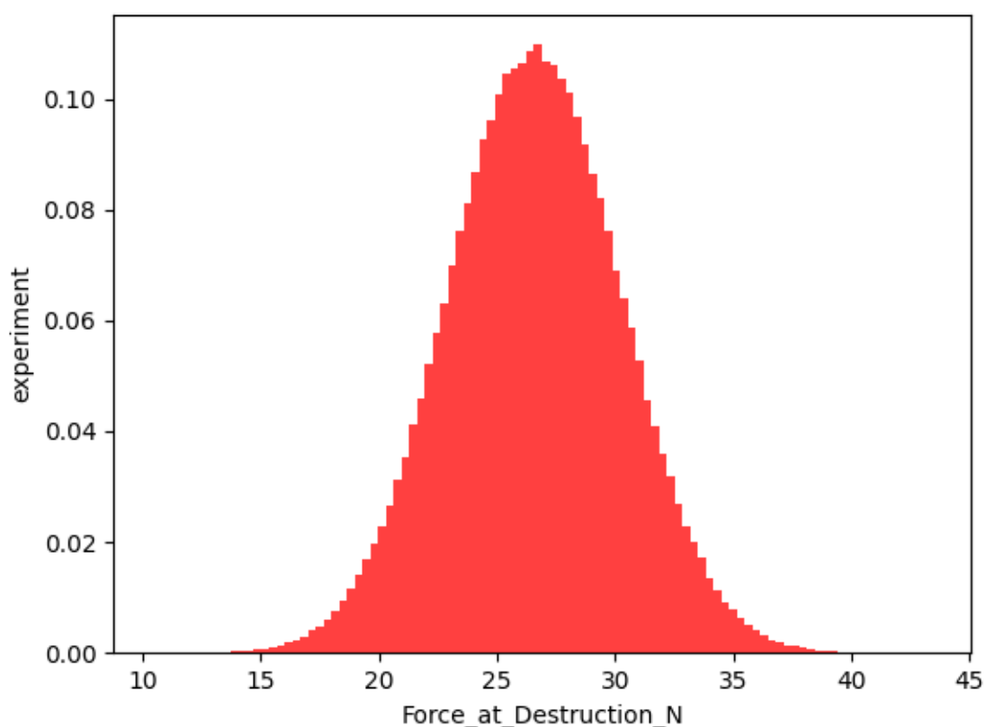
Рисунок 12. Нормальное распределение результатов измерения силы разрыва плёнки
