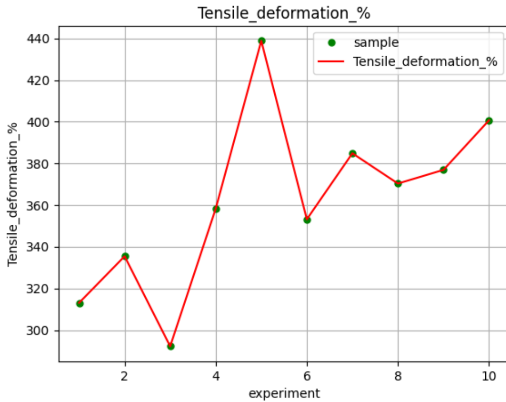
Рисунок 3. Деформация плёнки, %
