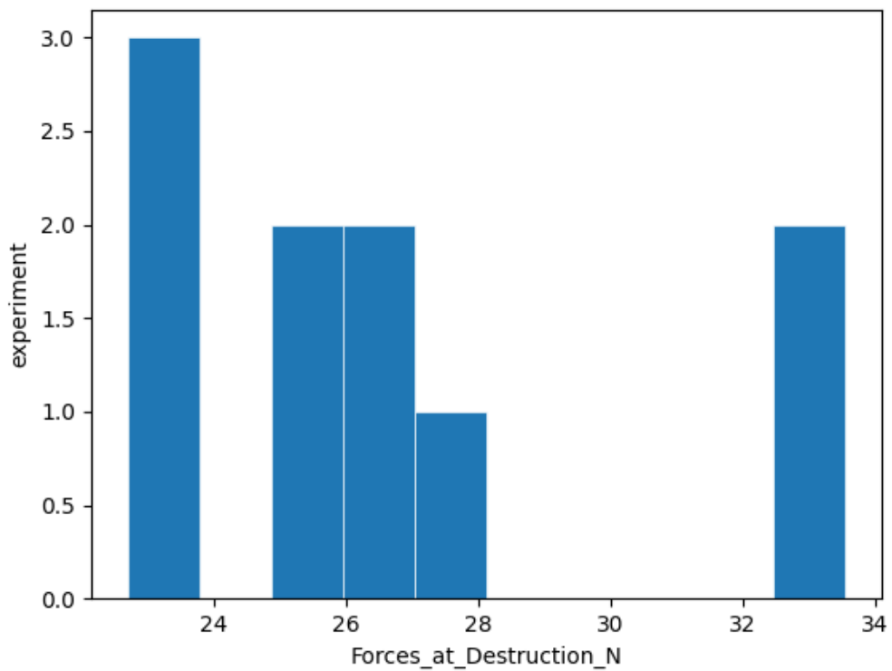
Рисунок 8. Распределение результатов измерения силы разрыва нити
