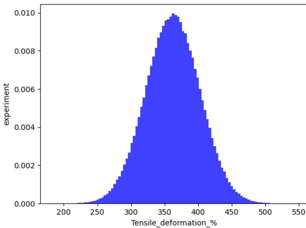
Рисунок 11. Нормальное распределение результатов измерения деформации плёнки
