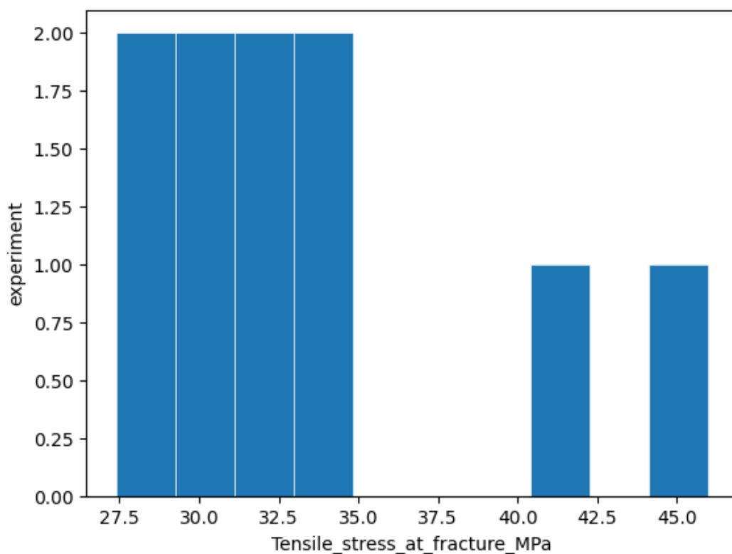
Рисунок 6. Распределение результатов измерения растягивающего напряжения
