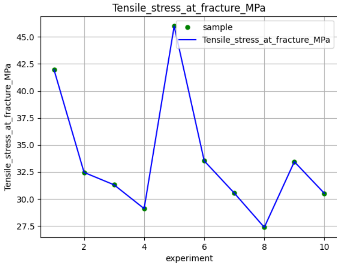
Рисунок 2. Растягивающее напряжение, МПа
