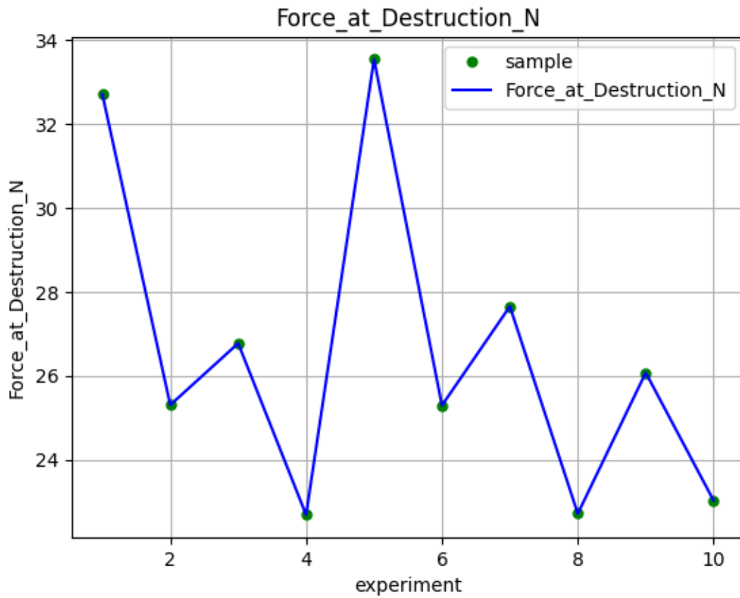
Рисунок 4. Сила разрыва плёнки, Н
