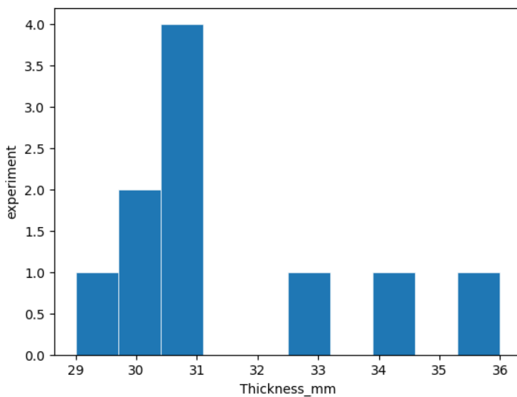
Рисунок 5. Распределение результатов измерения толщины плёнки
